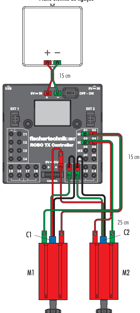
Schakelschema Diagrama de circuitos Plano elétrico de ligação
